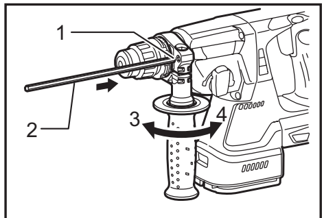
► 1. Hole 2. Depth gauge 3. Loosen 4. Tighten
